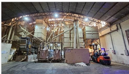
Galpão 2 | Fonte: GT
