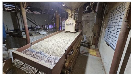
Catadores de pedras | Fonte: GT
